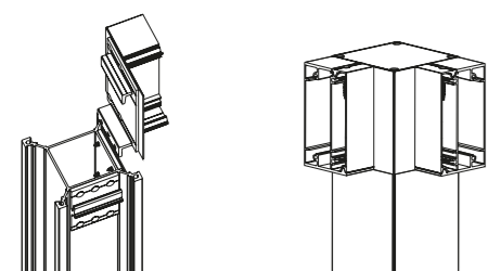
Σύνδεση κολόνας με τραβέρσα
