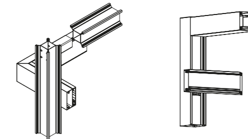
Σύνδεση προφίλ κολόνας και τραβέρσας
